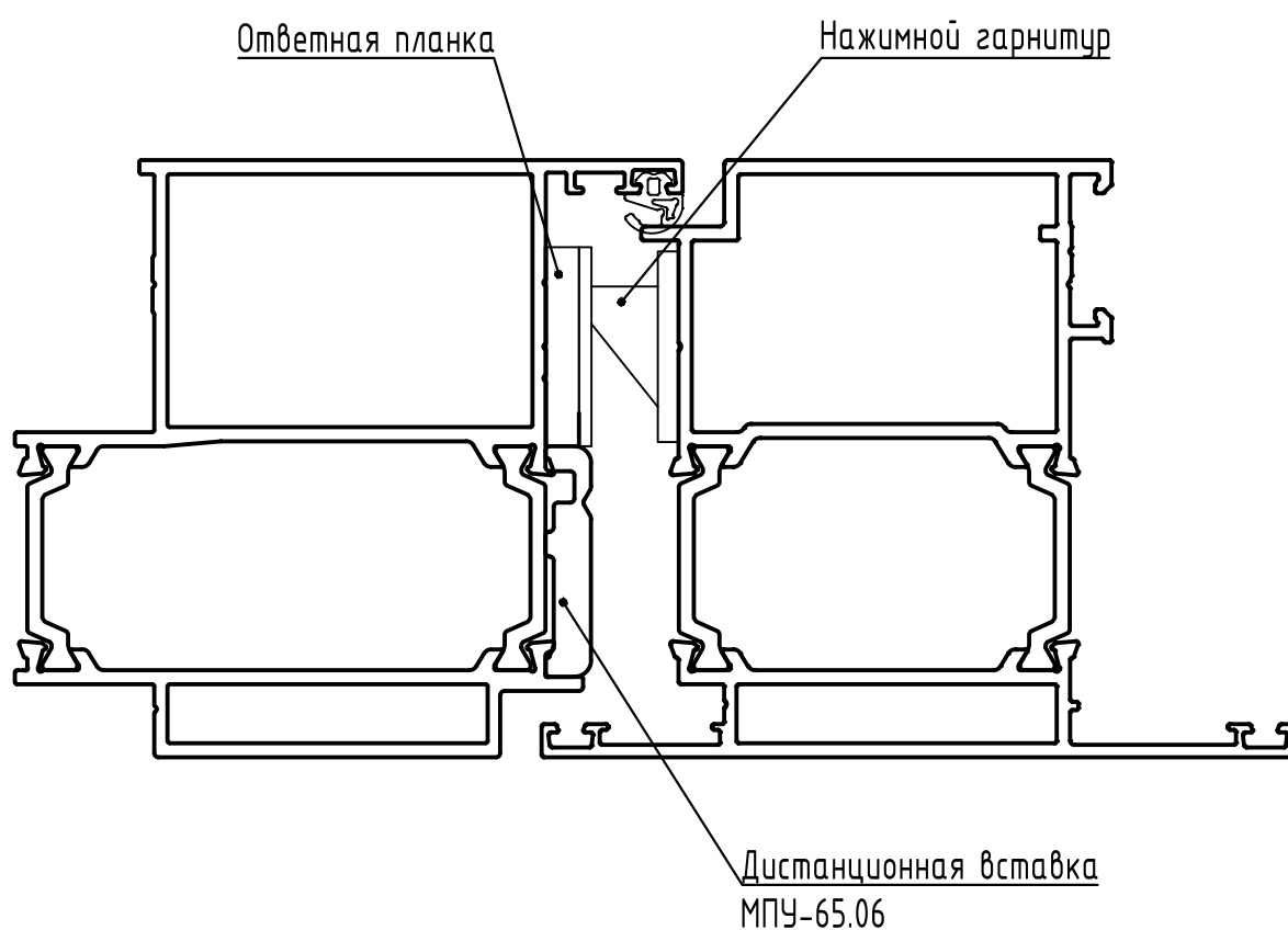
Установка МПУ-65.06 в дверях серии МП-72
